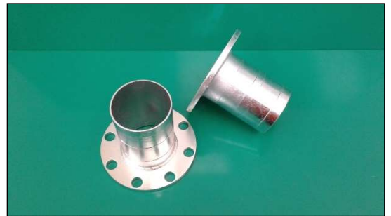
Portagomma flangiati. Tronchetto per tubo da 4".
